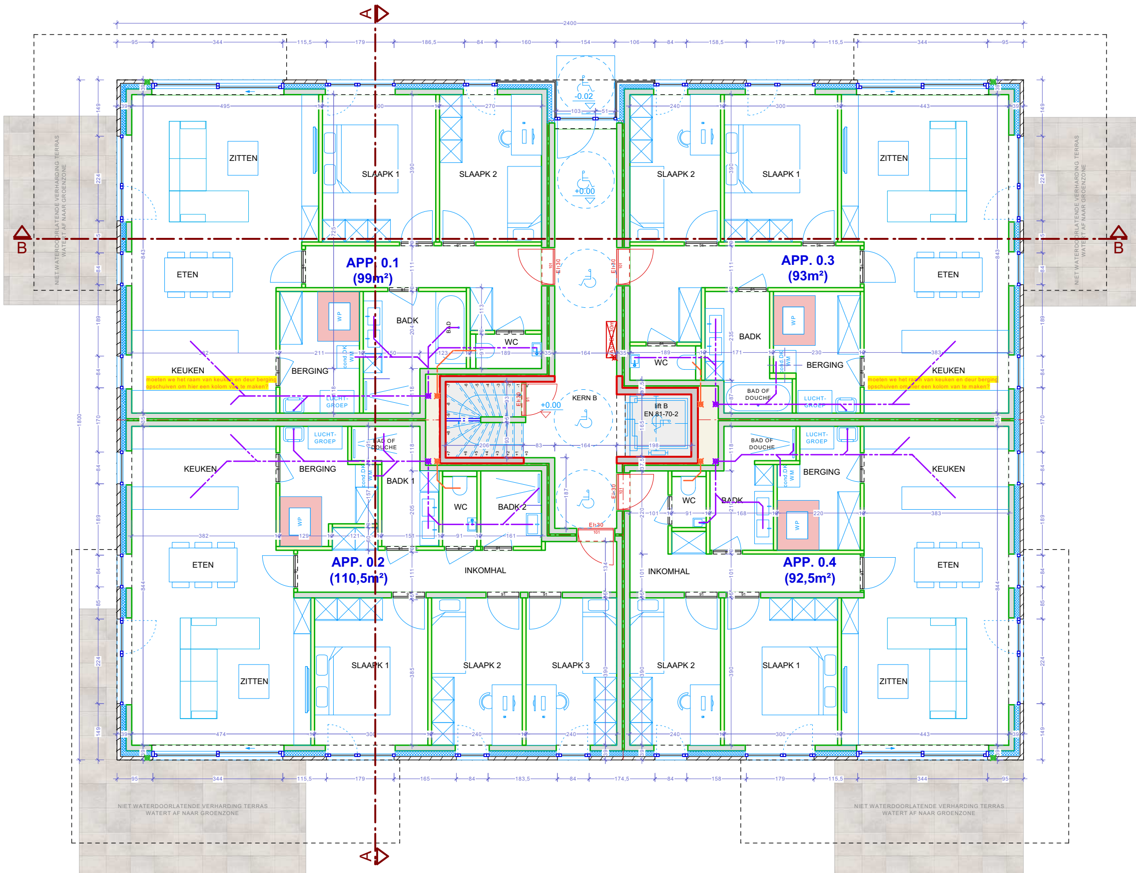
GEBOUW B - GELIJKVLOERS +0.00
