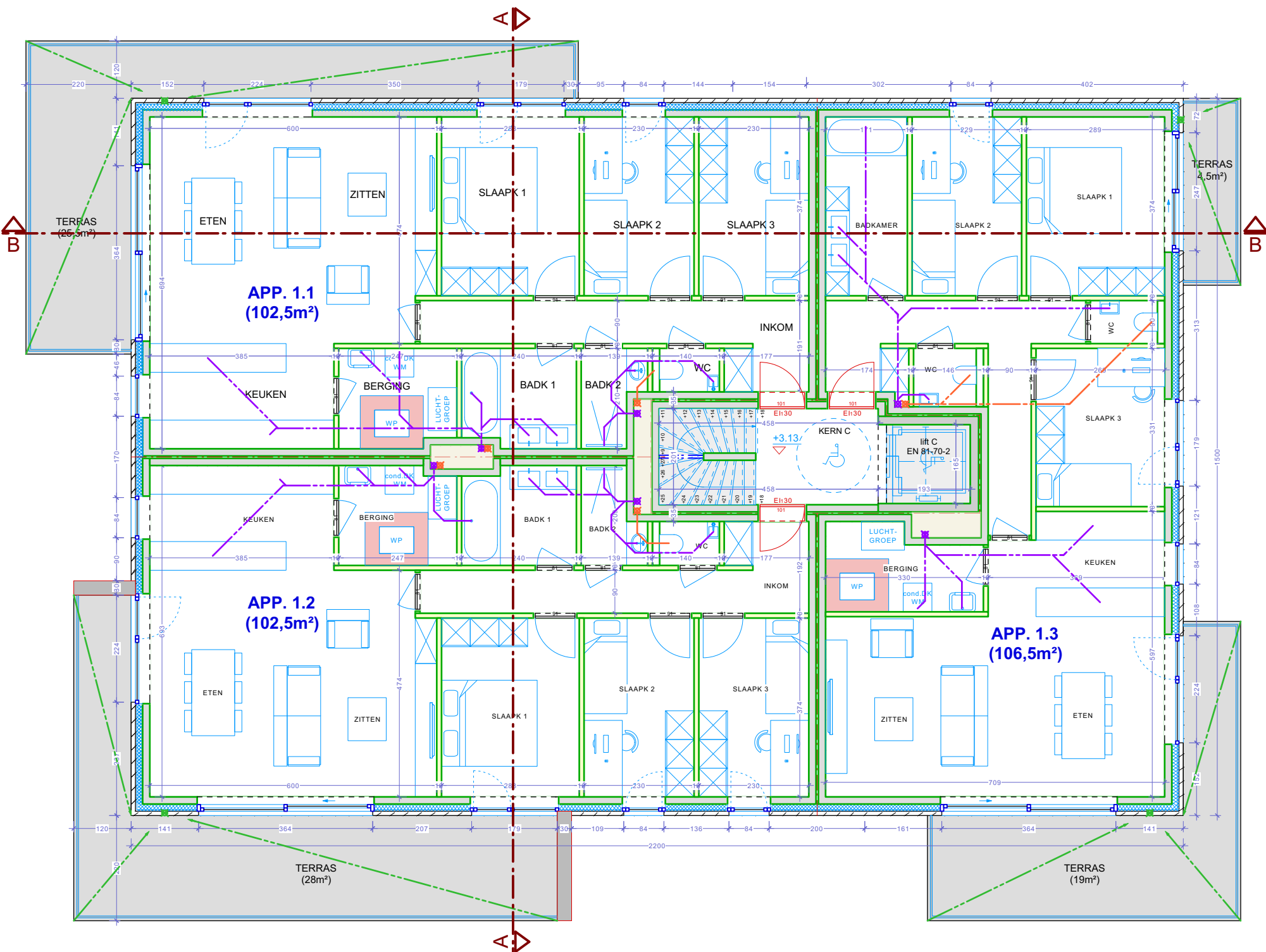
GEBOUW C - VERDIEPING +1
