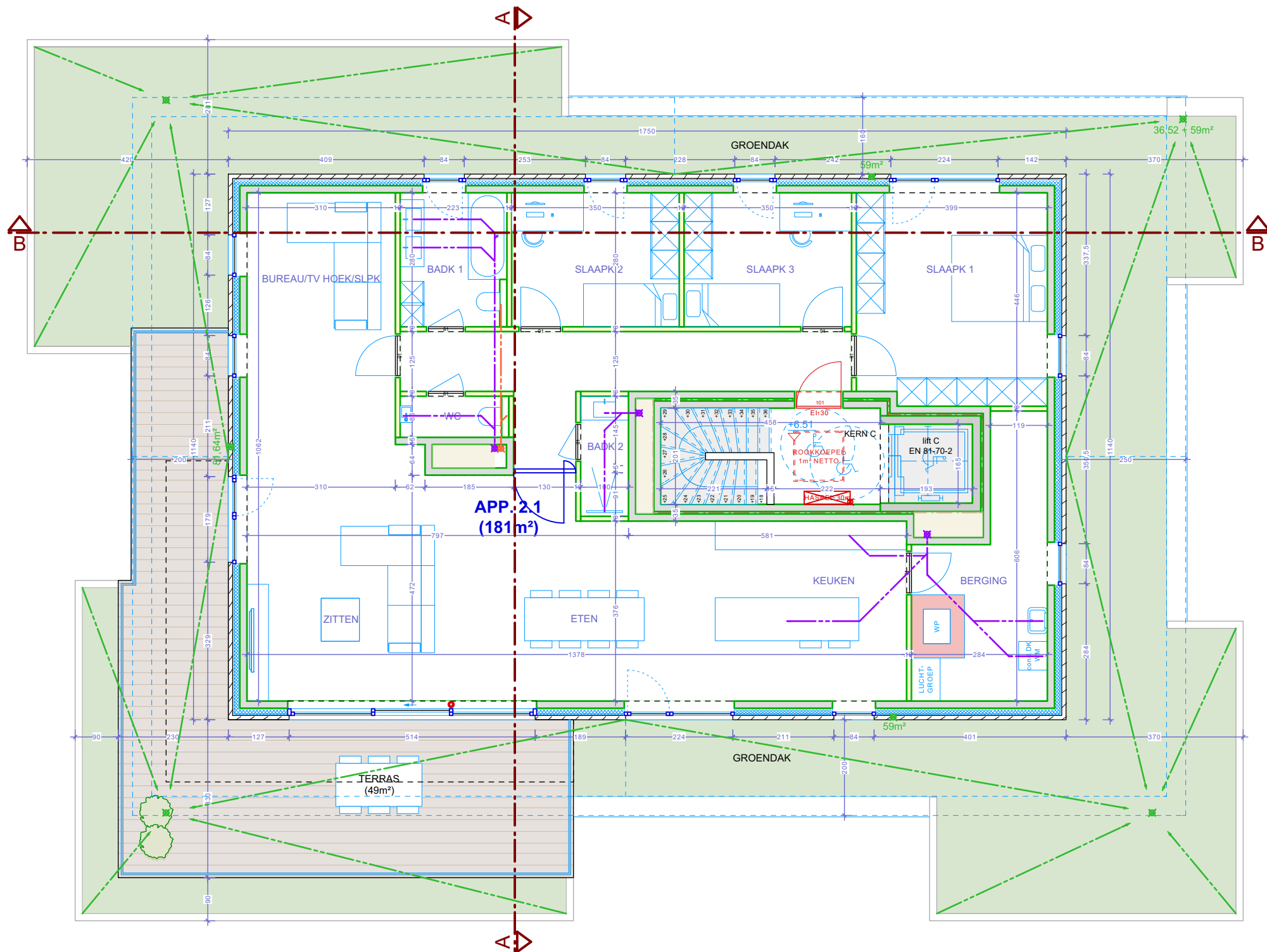
GEBOUW C - VERDIEPING +2
